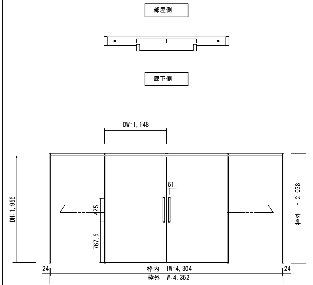
正面図
