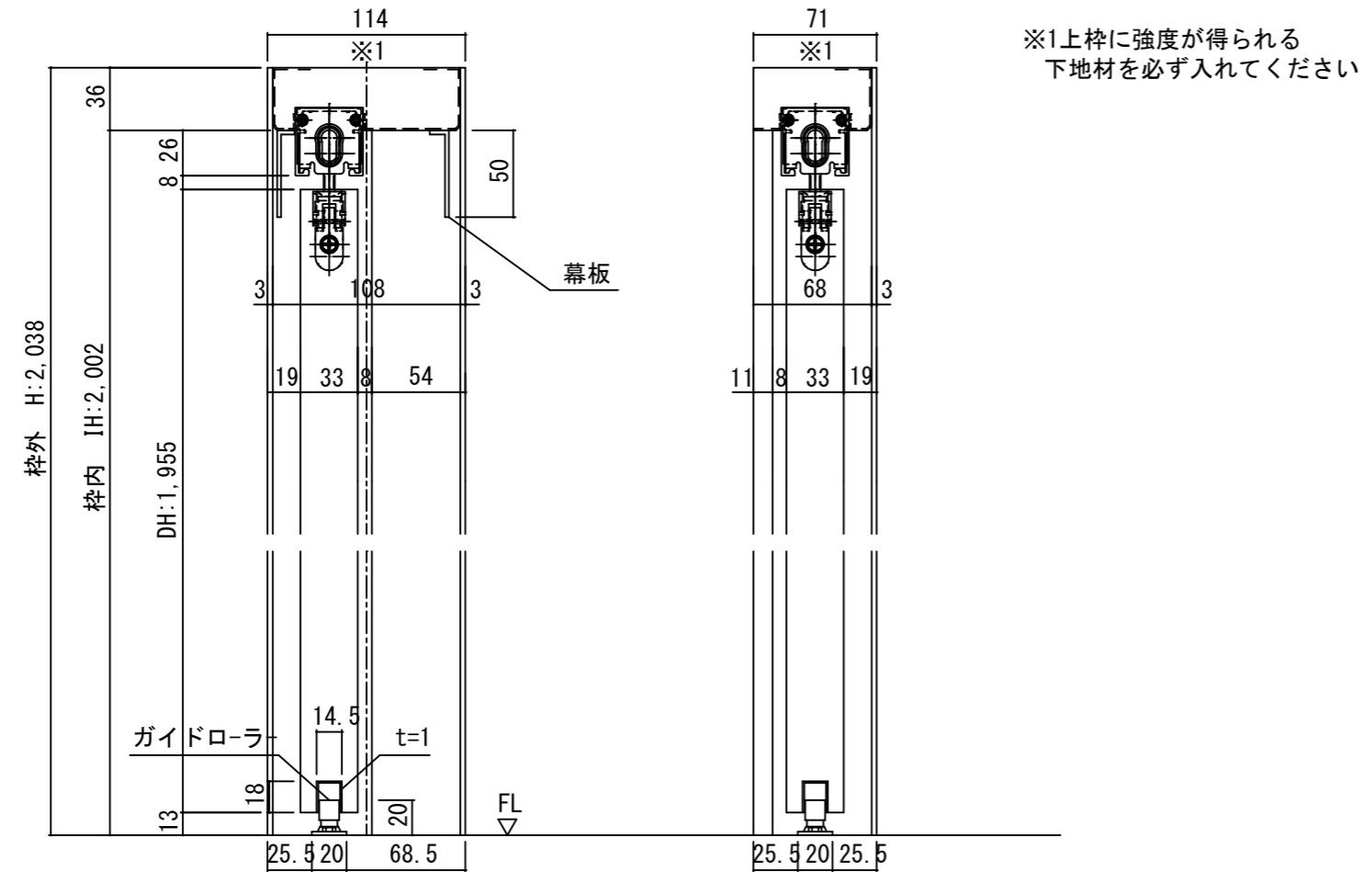
断面図
