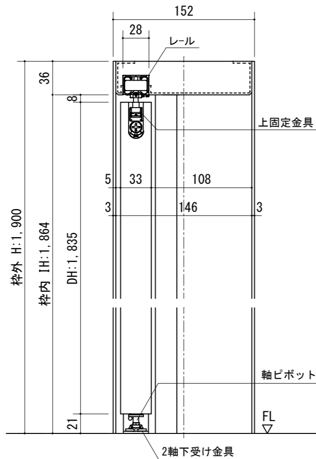
断面図
