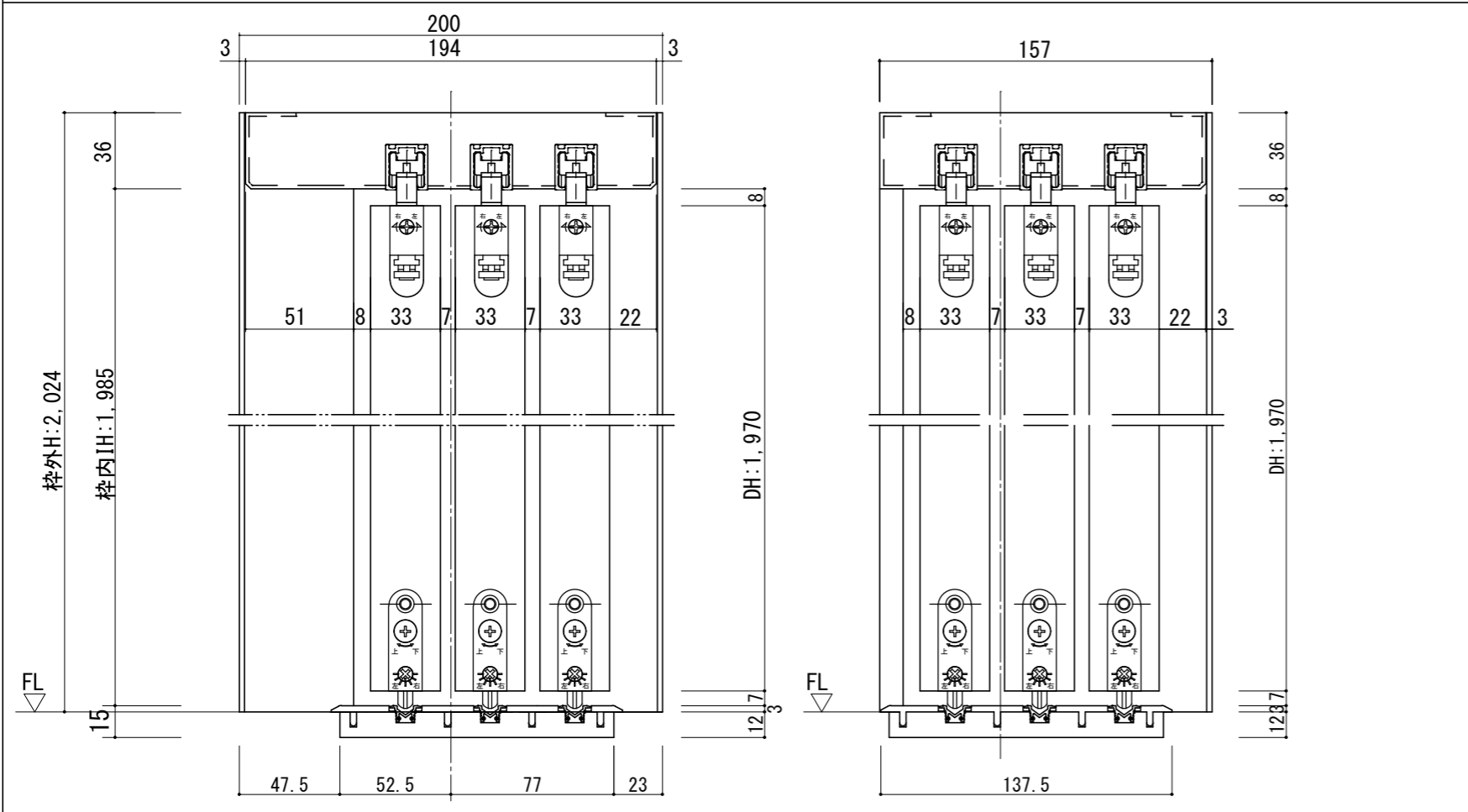
断面図
