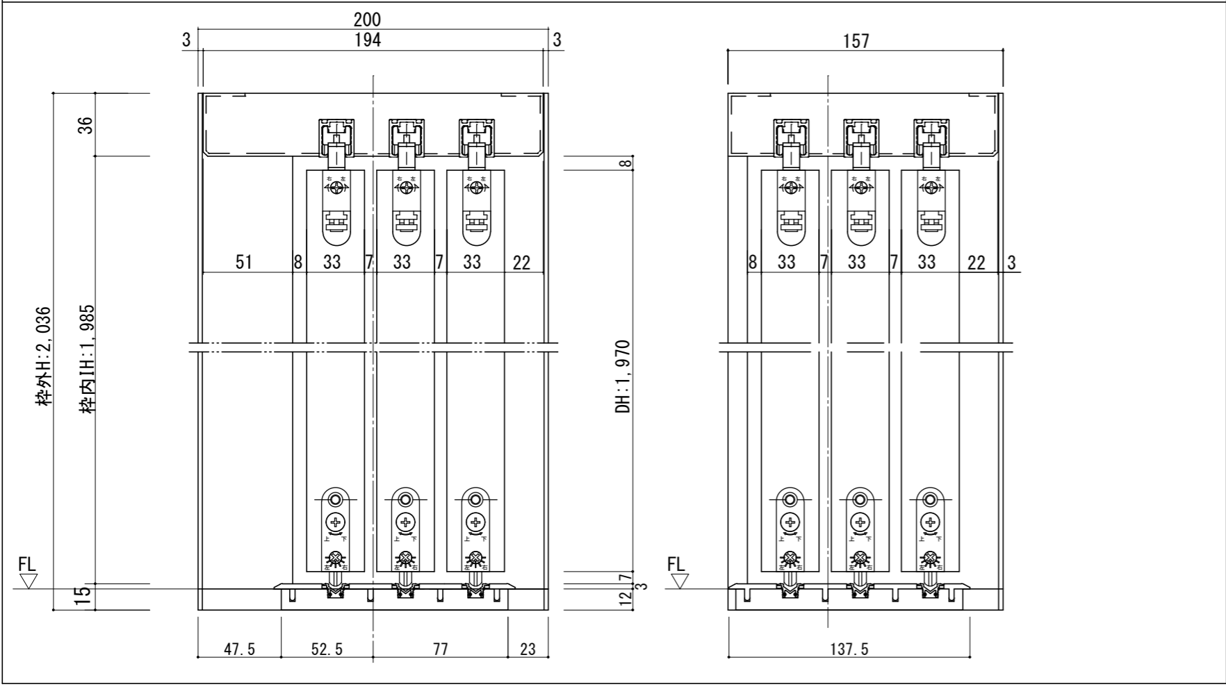
断面図
