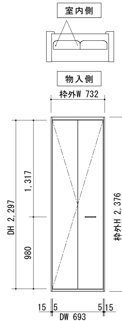
正面図
