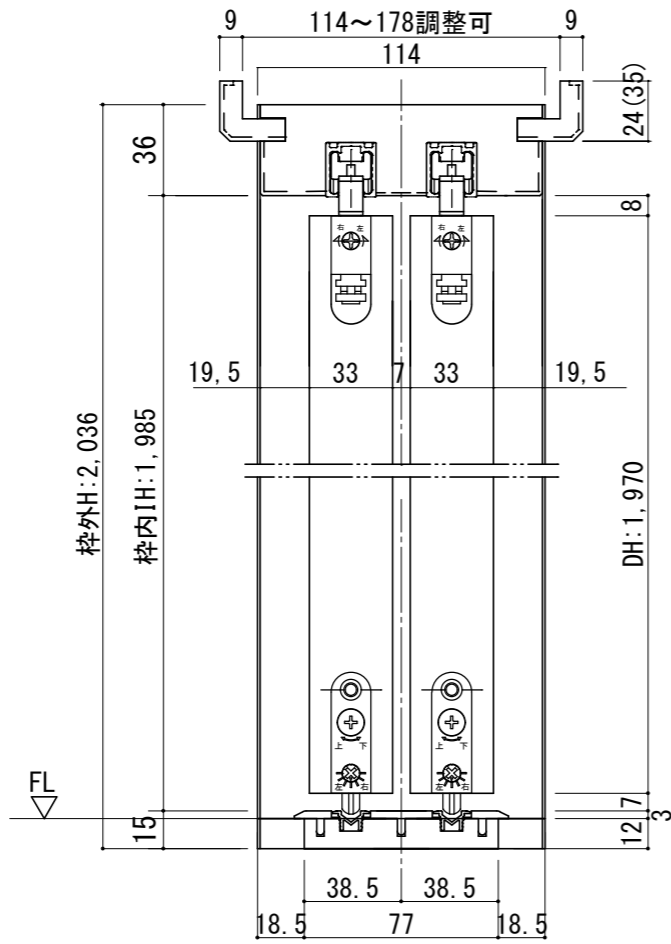
断面図
