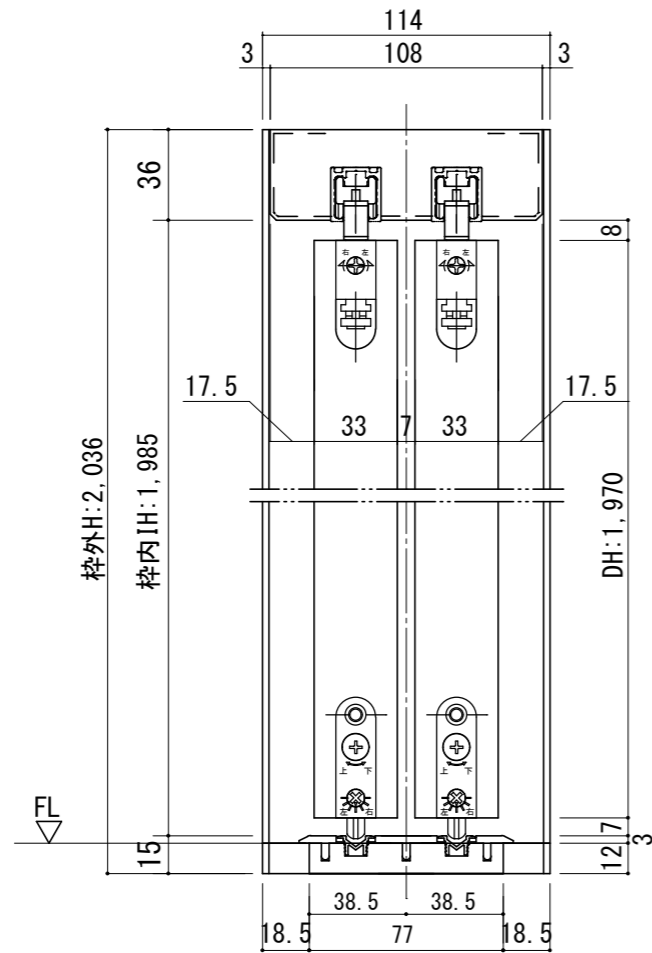
断面図
