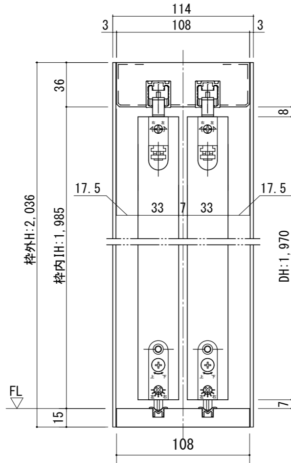
断面図
