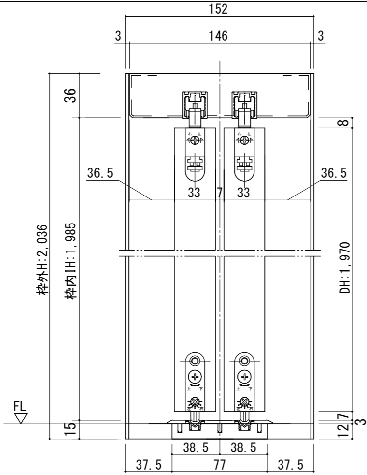
断面図
