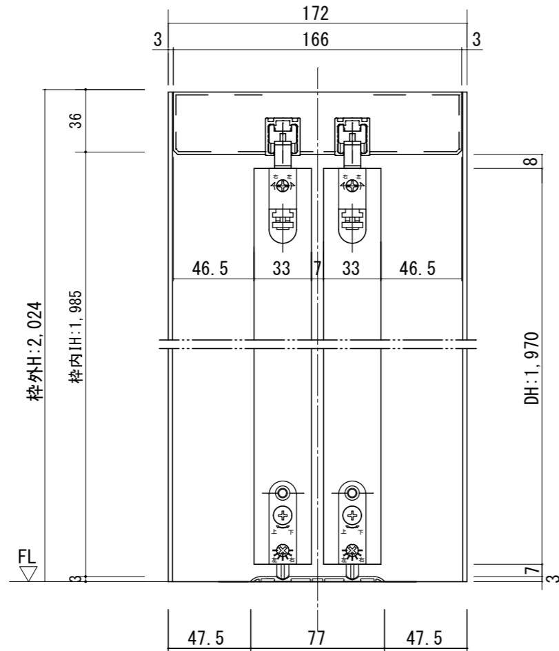
断面図
