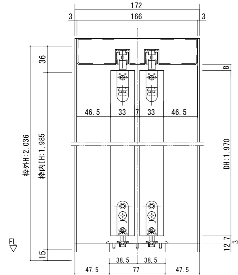
断面図
