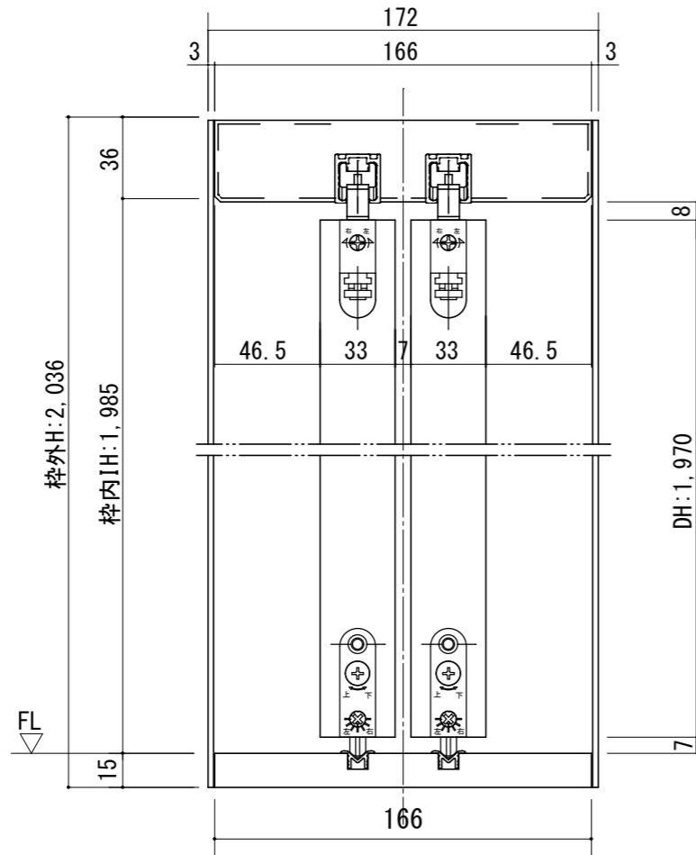
断面図
