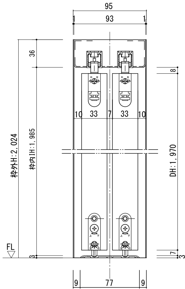
断面図
