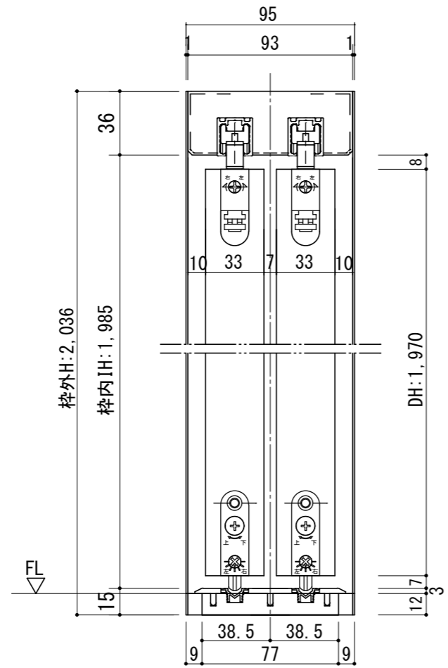
断面図
