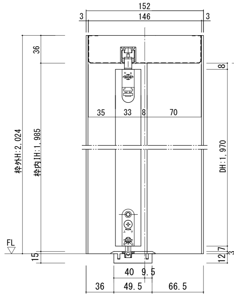
断面図
