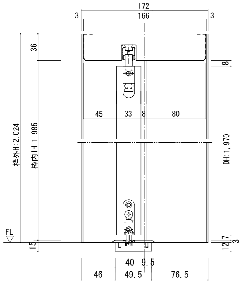
断面図
