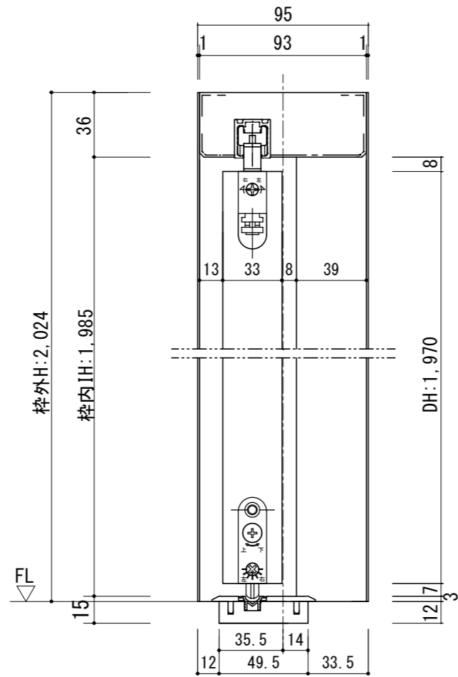
断面図
