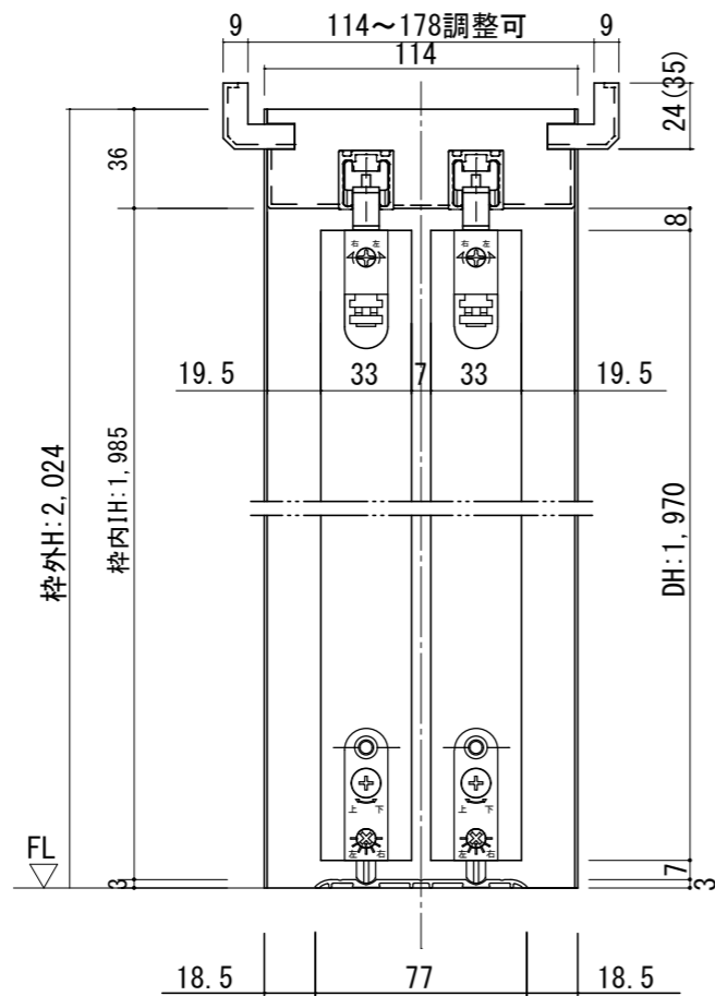
断面図
