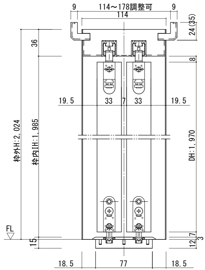
断面図
