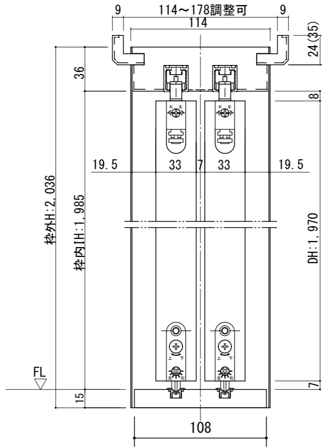
断面図
