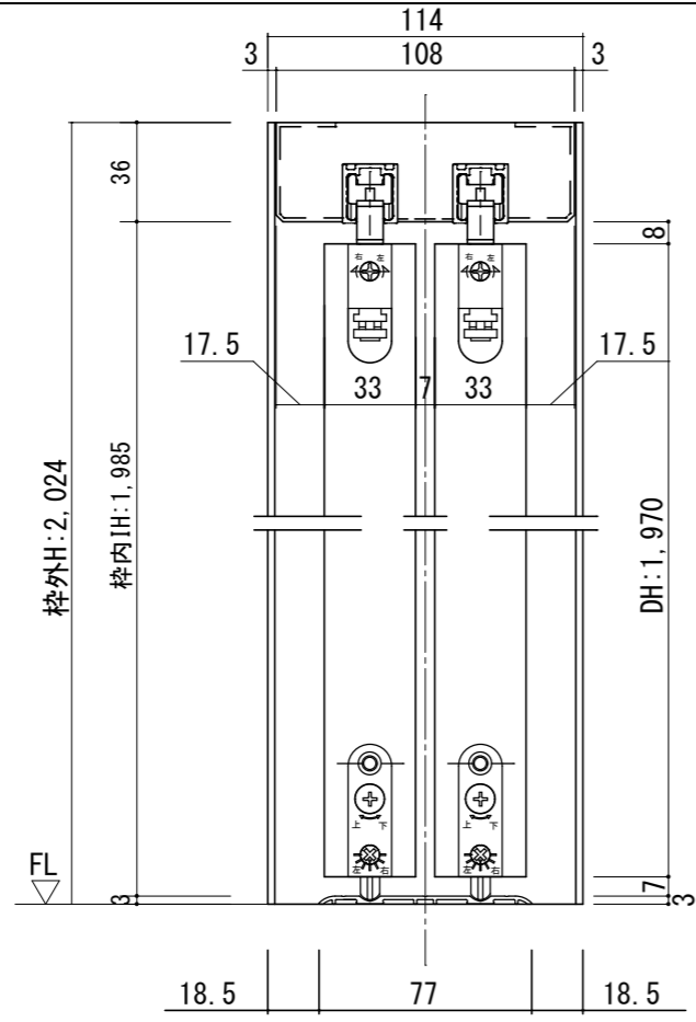
断面図
