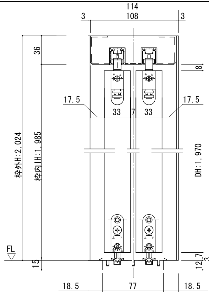
断面図
