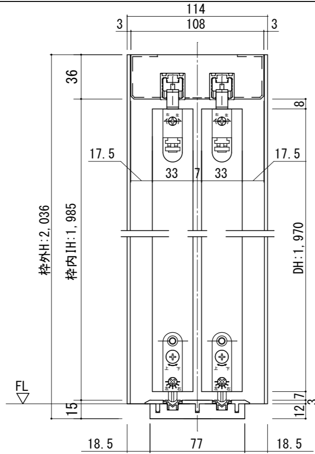
断面図
