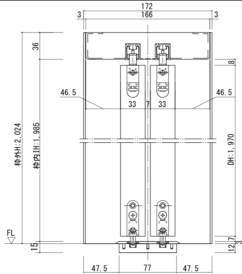
断面図
