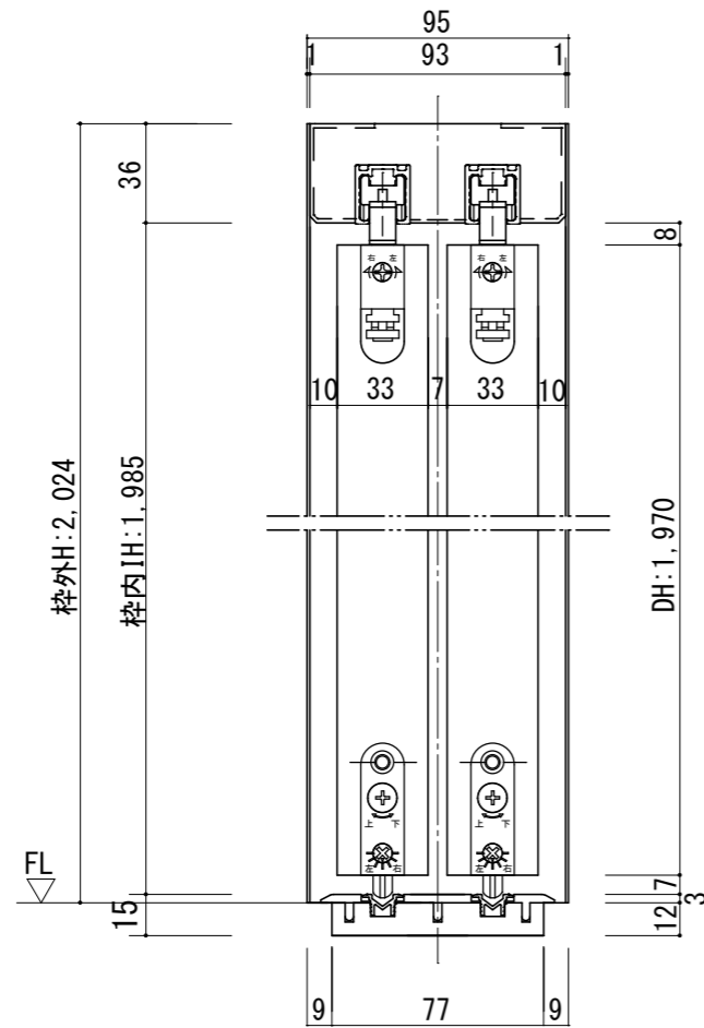
断面図
