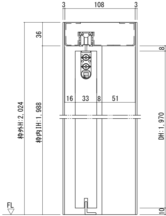
断面図
