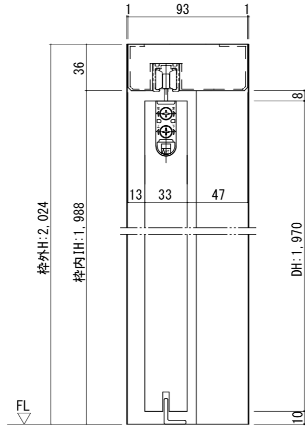
断面図
