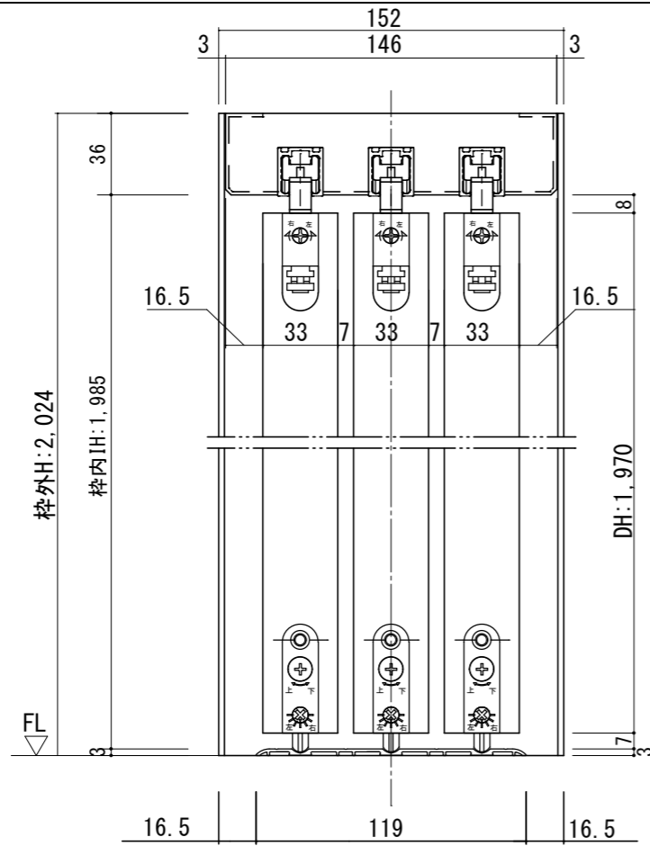
断面図
