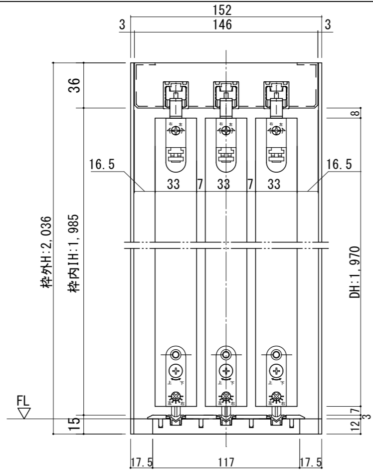
断面図
