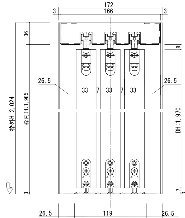
断面図
