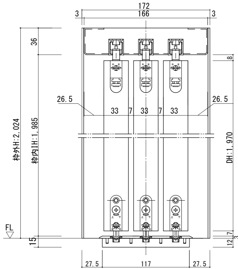
断面図
