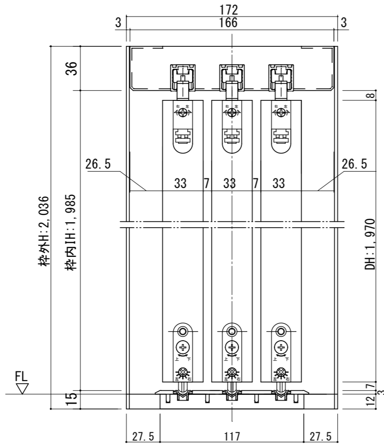
断面図
